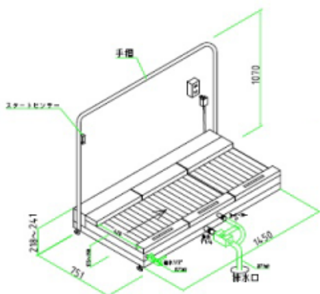
ピットソール3連式手摺仕様
