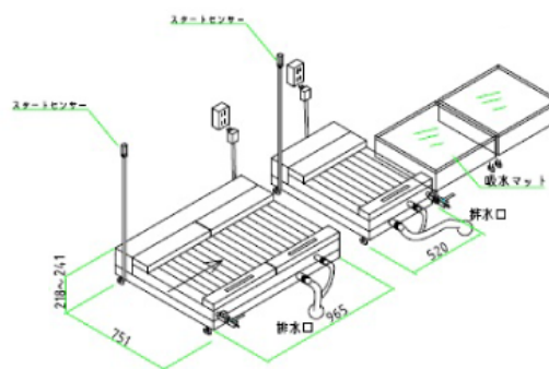
ピットソール2連式+標準機+給水台
